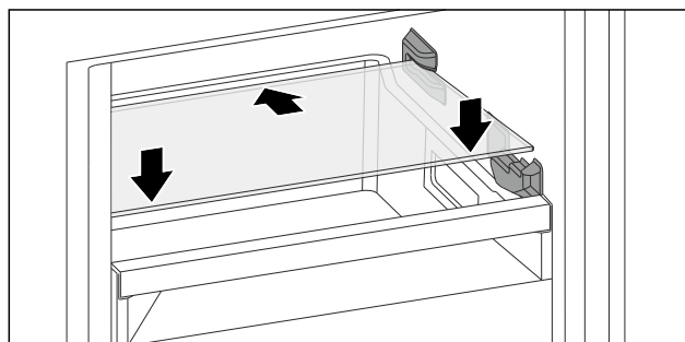
Fig. 121 Vejledende illustration af isætning af glasplade
